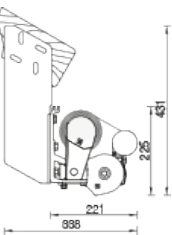
Installazione sottotetto
