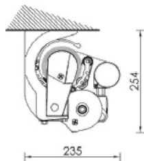
Installazione a soffitto
