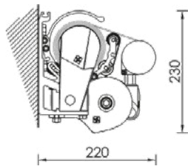
Installazione a parete
