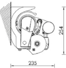
Installazione a parete con staffa universale
