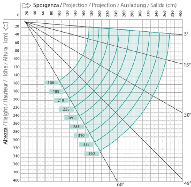
Diagramma di copertura a parete
